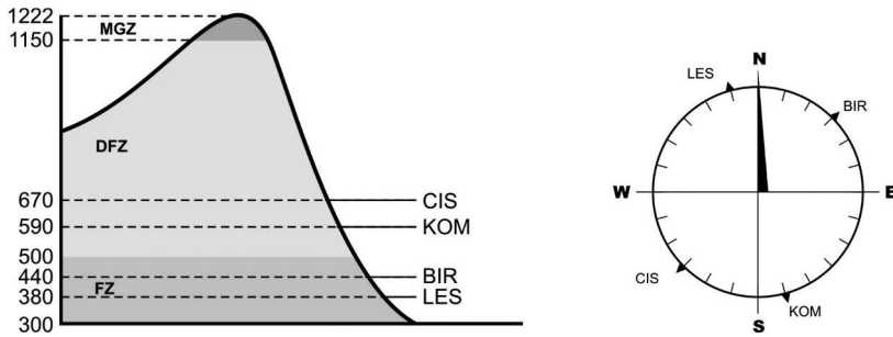
Rycina 3. Gradient wysokości i kierunków geograficznych wystawy powierzchni testujących. MGZ – piętro polonin, DFZ – piętro regla dolnego, FZ – piętro pogórza. Pozostałe oznaczenia jak na rycinie 2. Figure 3. Elevation gradient and geographical directions of exposure of experimental plots. MGZ – mountain grassland zone, DFZ – lower mountain deciduous forest zone, FZ – foothills zone. Other designation as in Figure 2.
