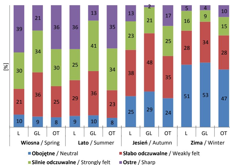
Rycina 5. Częstość [%] występowania bodźców termicznych wyznaczonych na podstawie wartości amplitudy temperatury powietrza, lata 2010–2011; L, GL, OT – jak na rycinie 1 Figure 5. Occurrence frequency [%] of thermal incentives calculated based on differences of daily maximal and minimal air temperature in 2010–2011; L, GL, OT – as in Figure 1.
