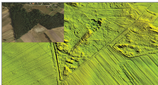
Ryc. 3. Obiekt rozpoznany na podstawie ALS (niezidentyfikowany wcześniej), z charakterystycznymi zniszczeniami, związanymi z nielegalnym pozyskiwaniem piasku. Regionalna Dyrekcja Lasów Państwowych w Poznaniu, Nadleśnictwo Koło (MGGP Aero / oprac. R. Zapłata).
