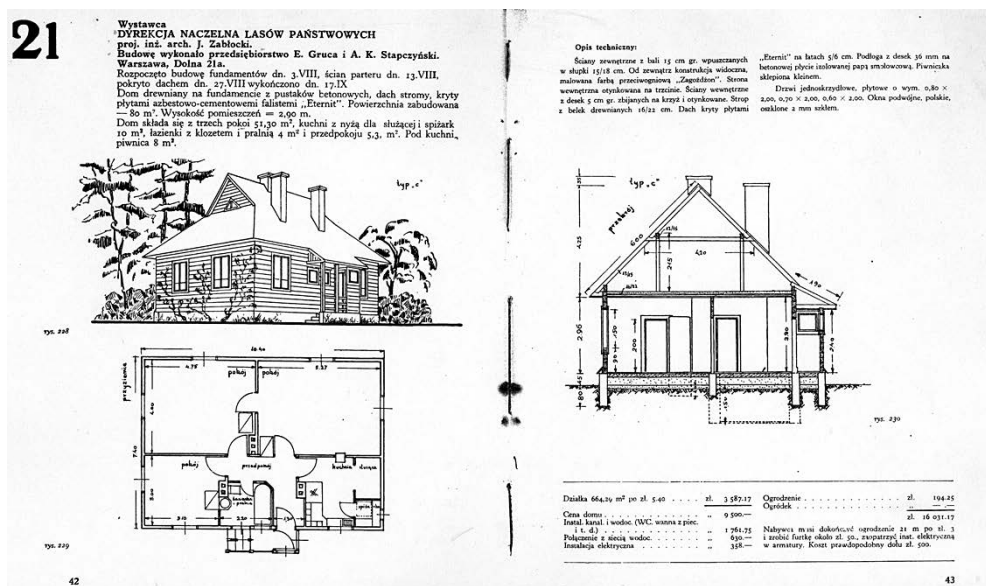
Ryc. 17. Katalog Wystawy Tani Dom Własny (1932) – projekt trzypokojowego drewnianego domu mieszkalnego wystawionego przez Dyрекcję Naczelną Lasów Państwowych. Proj. inż. arch. J. Zabłocki (ok. 1932). Wg „Dom-Osiedle-Mieszkanie” 1932. Nr 7–8.
