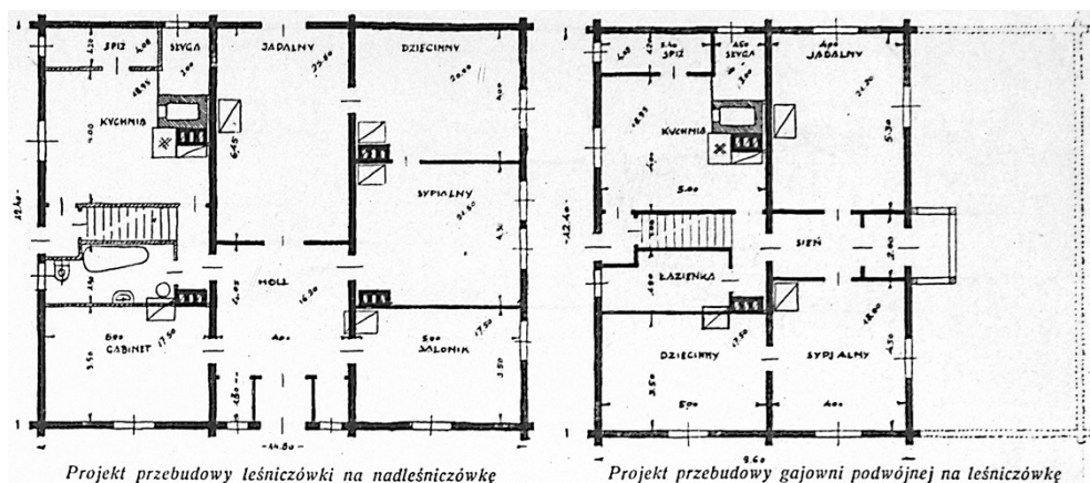
Ryc. 16. Plany typowych: nadleśniczówki, leśniczówki i podwójnej gajówki. Proj. J. Zabłocki [?] (ok. 1930). Wg „Echa Leśne”, 1930, nr 12.
