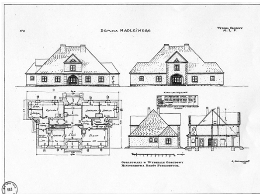
Ryc. 3. Projekt wzorcowy drewnianego domu dla nadleśniczego Nr 1. Proj. R. Gutt (1919). Wg „Odbudowa Kraju. Projekty domów dla dozoru leśnego”. Wyd. Wydziału Odbudowy MRP (ok. 1920).
