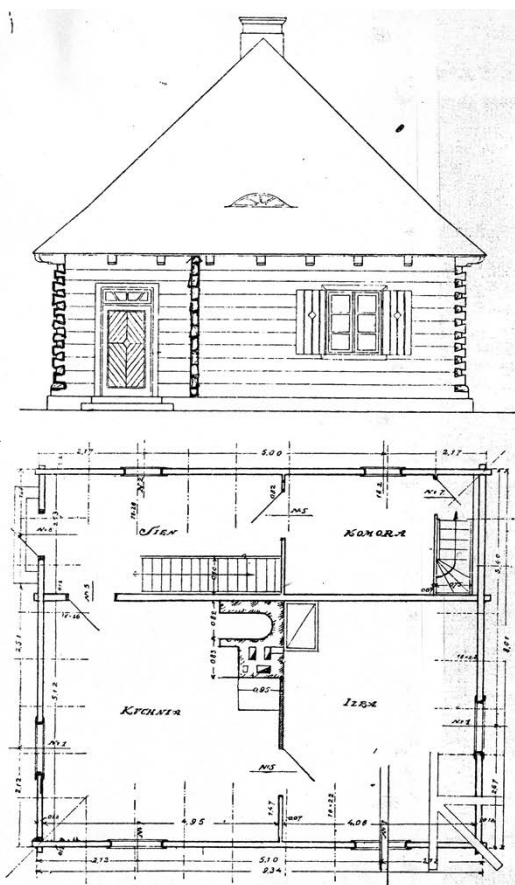
Ryc. 5. Projekt drewnianej gajówki zatwierdzony do realizacji przez Ministerstwo Rolnictwa – plan przyziemia i elewacja frontowa. Proj. M. Kontkiewicz (ok. 1924). Wg S. Turczynowicz, „Budowle wiejskie...”, Warszawa (1927)
