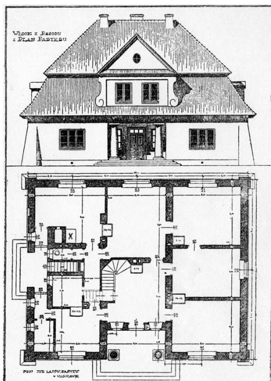
Ryc. 6. Projekt murowanej nadleśniczówki opracowany na zlecenie Dyrekcji Lasów Państwowych – plan parteru i piętra oraz elewacja frontowa i boczna. Proj. K. Modliński (ok. 1925). Wg S. Turczynowicz, „Budowle wiejskie...”, Warszawa (1927).
