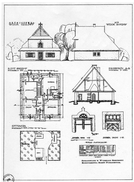
Ryc. 4. Projekt wzorcowy leśniczówki murowanej Nr 4 (ok. 1919). Wg „Odbudowa Kraju. Projekty domów dla dozoru leśnego”. Wyd. Wydziału Odbudowy MRP (ok. 1920).
