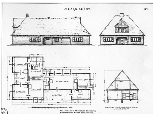
Ryc. 2. Projekt wzorcowy drewnianego budynku urzędu leśnego Nr 4 (ok. 1919). Wg „Odbudowa Kraju. Projekty domów dla dozoru leśnego”. Wyd. Wydziału Odbudowy MRP (ok. 1920).
